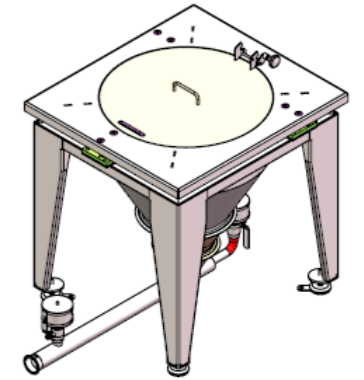
• Trémie équipée de peson
