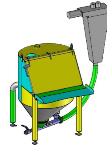
• Vide sac avec aiguillage
